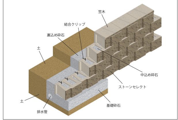
標準施工断面図（重力式工法）
