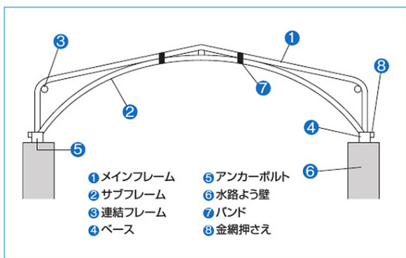
エコプロガードの構造
