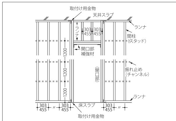
壁下地 組付図
