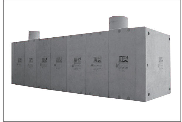
狭隘な場所で施工できるようにブロックを6tトラックで搬入可能にした狭隘型貯水槽
