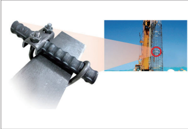
無溶接金具 KSクルリン
