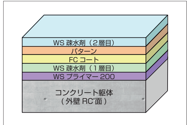
FC 特殊工法塗装時のモデル図
