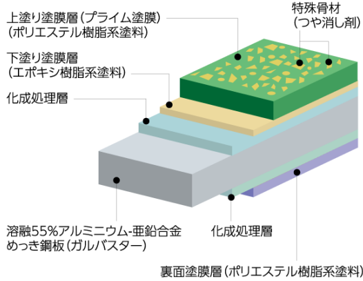
セリオス・プライムの構造
