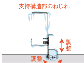
SZ-ADの高さ調整機能
