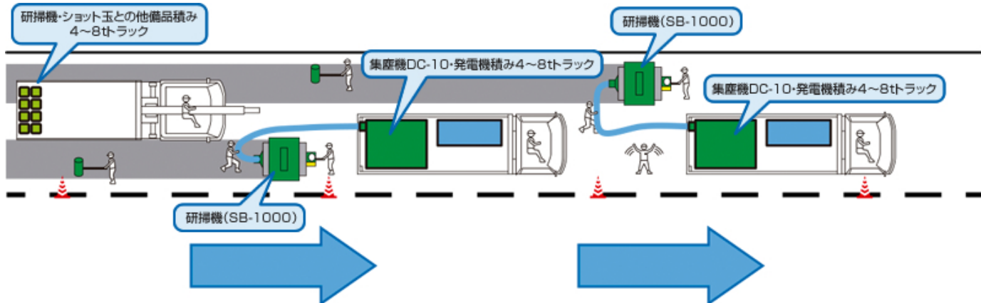
トンネル内コンクリート舗装面のギガショット (施工配置図)
