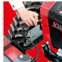
③ 電気デバイスのコネクターを抜く
