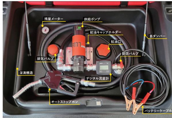
容器構造 (mobiFITT190L)
