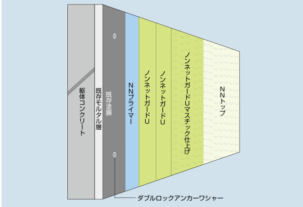
ノンネットガードU-M工法 (モルタル塗り外壁) 施工イメージ
