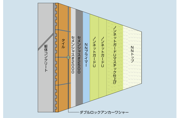
ノンネットガードU-T工法 (タイル張り外壁) 施工イメージ
