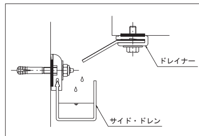
橋梁伸縮ジョイント部排水装置
