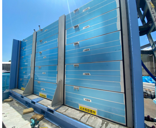
脱着式止水板 (高水圧用) 設計水深2.5mまで対応 WS-6相当
