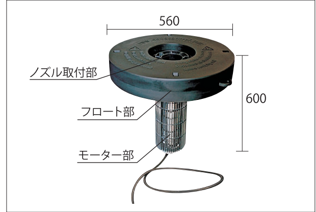
本体写真
