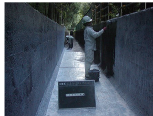
③プライマー塗布
