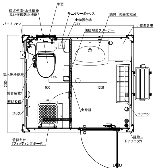
ブリリアントS (1個室タイプ) 平面図
