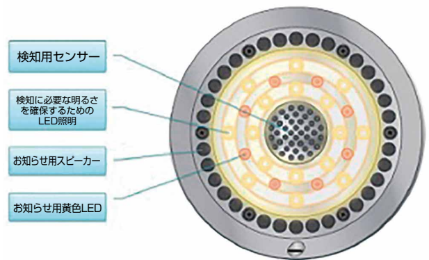
センサー詳細図 (直径約15cm)
